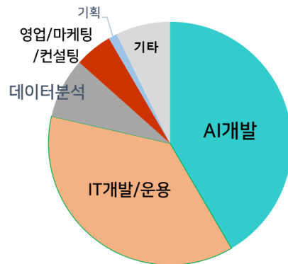
[AI개발자트랙]
