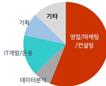
[DX컨설턴트 트랙]
